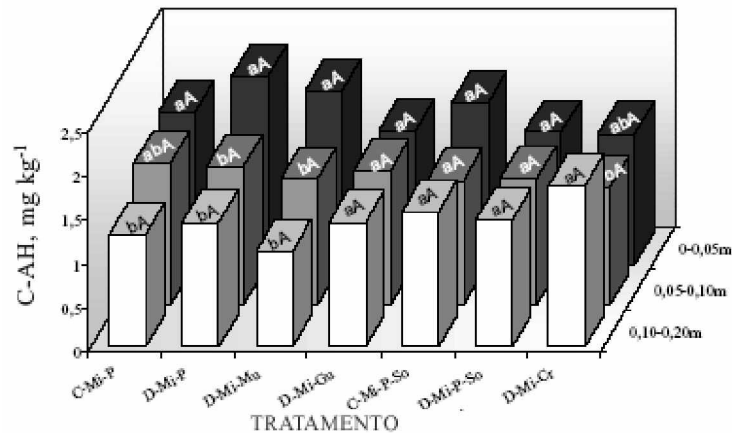
Figura 4. Teores de carbono na fração ácido húmico em um Latossolo Roxo com milho sob diferentes sistemas de produção por seis anos. C = sistema de semeadura convencional; D = sistema plantio direto; Mi = milho semeado no verão; So = soja semeada no verão; P = pousio no inverno; Mu = semeadura de mucuna preta no inverno; Gu = semeadura de feijão guandu no inverno; Cr = semeadura de crotalária no inverno. Médias seguidas de mesma letra não diferem entre si pelo Teste de Tukey, a 5 %. Letras minúsculas comparam médias dispostas na vertical. Letras maiúsculas comparam médias dispostas na horizontal.
