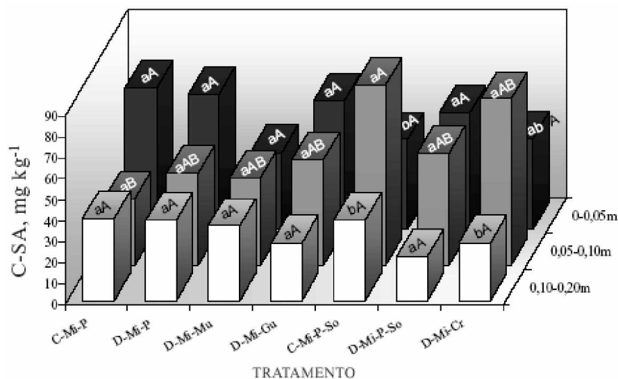
Figura 1. Teores de carbono solúvel em água em um Latossolo Roxo cultivado com milho sob diferentes sistemas de produção por um período de seis anos. C = sistema de semeadura convencional; D = sistema plantio direto; Mi = milho semeado no verão; So = soja semeada no verão; P = pousio no inverno; Mu = semeadura de mucuna preta no inverno; Gu = semeadura de feijão guandu no inverno; Cr = semeadura de crotalária no inverno. Médias seguidas de mesma letra não diferem entre si pelo Teste de Tukey, a 5 %. Letras minúsculas comparam médias dispostas na vertical. Letras maiúsculas comparam médias dispostas na horizontal.
