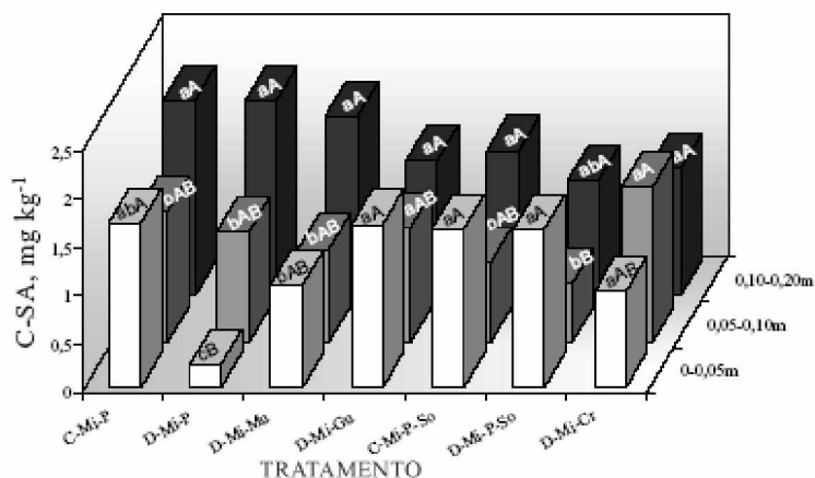
Figura 3. Teores de carbono na fração ácido fúlvico em um Latossolo Roxo cultivado com milho sob diferentes sistemas de produção por seis anos. C = sistema de semeadura convencional; D = sistema plantio direto; Mi = milho semeado no verão; So = soja semeada no verão; P = pousio no inverno; Mu = semeadura de mucuna preta no inverno; Gu = semeadura de feijão guandu no inverno; Cr = semeadura de crotalária no inverno. Médias seguidas de mesma letra não diferem entre si pelo Teste de Tukey, a 5 %. Letras minúsculas comparam médias dispostas na vertical. Letras maiúsculas comparam médias dispostas na horizontal.
