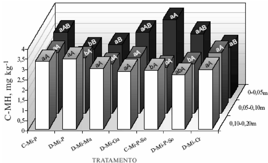
Figura 2. Teores de carbono solúvel em álcali (matérias húmicas), em um Latossolo Roxo cultivado com milho sob diferentes sistemas de produção por seis anos. C = sistema de semeadura convencional; D = sistema plantio direto; Mi = milho semeado no verão; So = soja semeada no verão; P = pousio no inverno; Mu = semeadura de mucuna preta no inverno; Gu = semeadura de feijão guandu no inverno; Cr = semeadura de crotalária no inverno. Médias seguidas de mesma letra não diferem entre si pelo Teste de Tukey, a 5 %. Letras minúsculas comparam médias dispostas na vertical. Letras maiúsculas comparam médias dispostas na horizontal.
